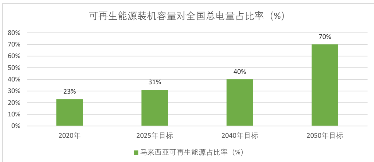
图 2-1 马来西亚可再生能源装机容量占全国总电量占比目标
